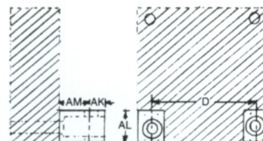
END LUG MOUNTS
